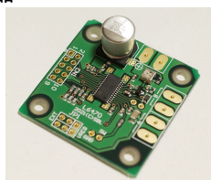
L6470 ドライバ基板
