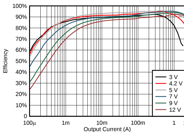
効率と出力電流との関係、 V_o = 5V
